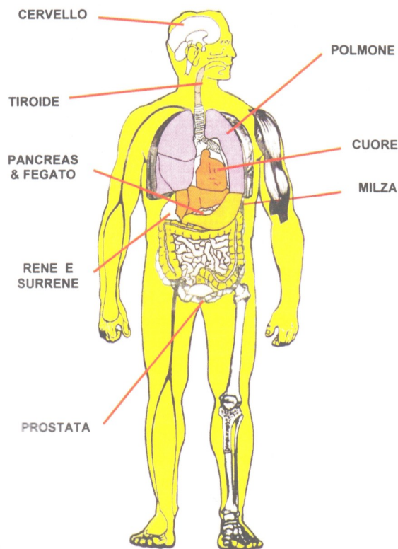
Fig. 1— Localizzazione dei corpuscoli dell'asbesto di lavoratori esposti
